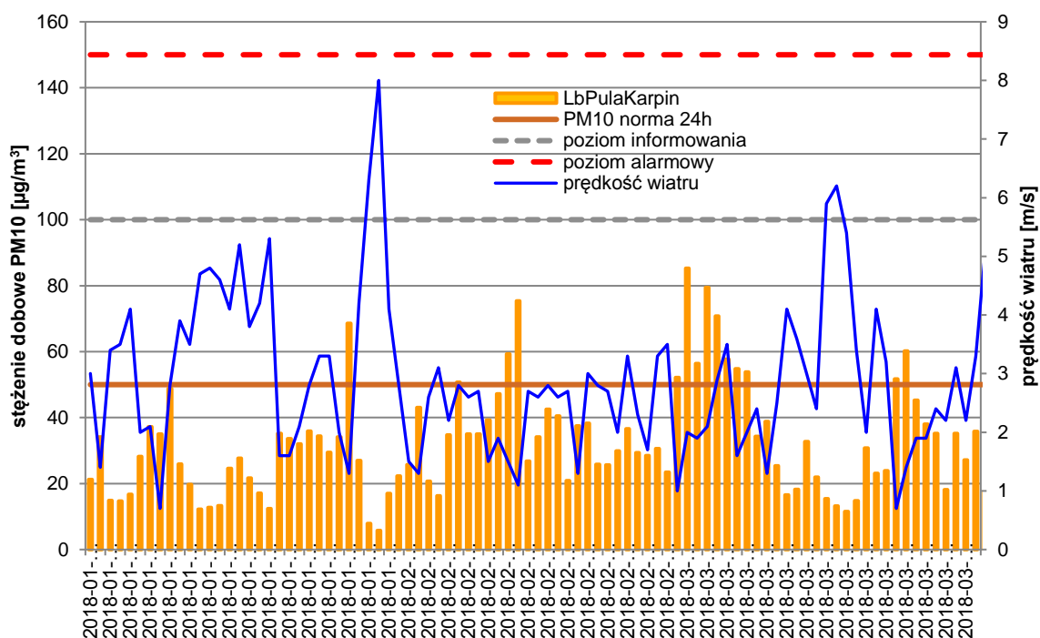
Rysunek 6. Przebieg zmienności stężeń 24-godz. PM10 w 2018 r. oraz prędkości wiatru w pierwszym kwartale 2018 roku w strefie lubelskiej w Puławach 45
