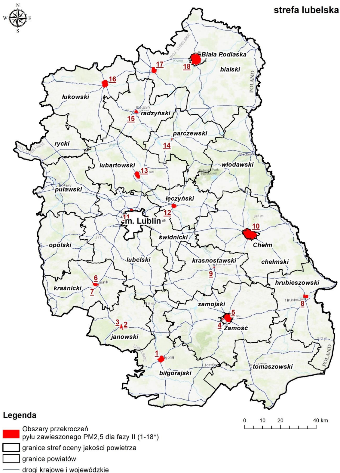
Rysunek 10. Obszary przekroczeń poziomu dopuszczalnego dla pyłu PM 2,5 na terenie strefy lubelskiej w 2018 roku 53
