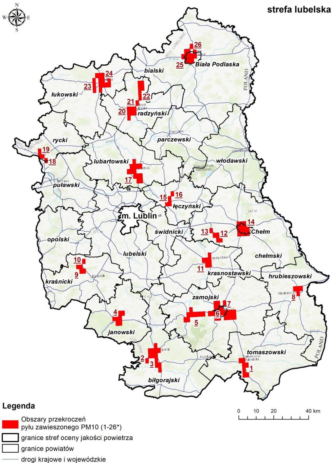
Rysunek 9. Obszary przekroczeń poziomu dopuszczalnego dla pyłu PM10 na terenie strefy lubelskiej w 2018 roku 52
