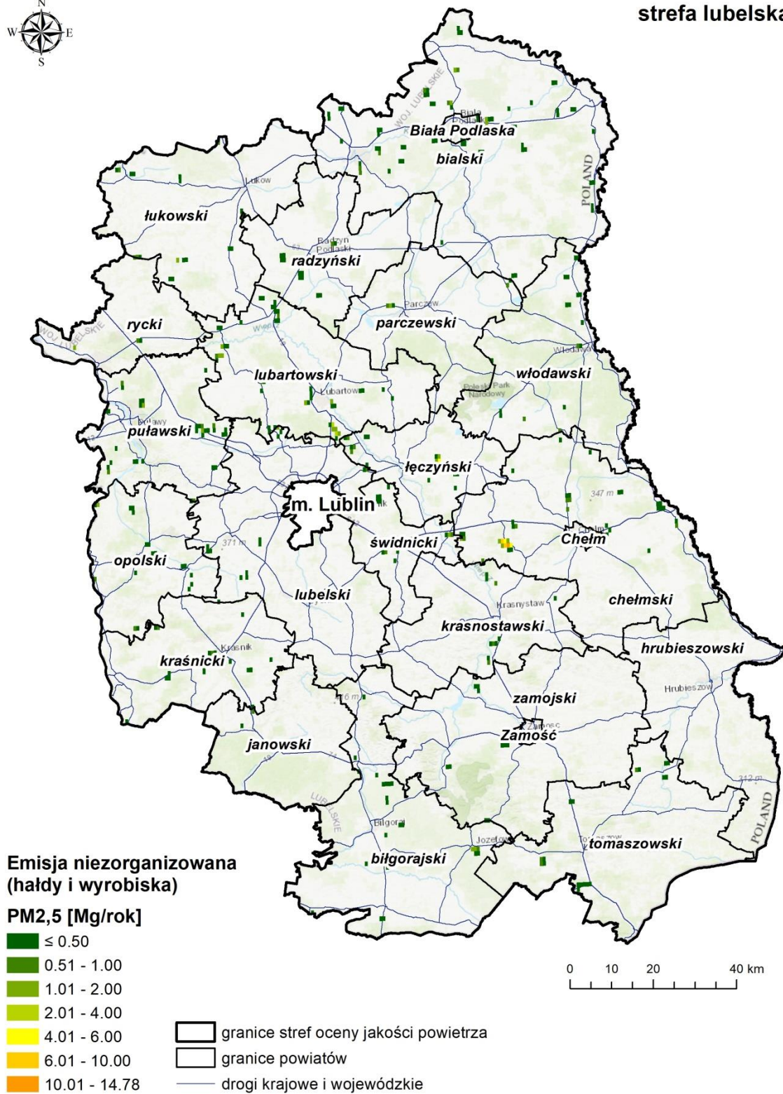
Rysunek 36. Emisja pyłu zawieszonego PM 2,5 ze źródeł niezorganizowanych (hałdy i wyrobiska) 98
