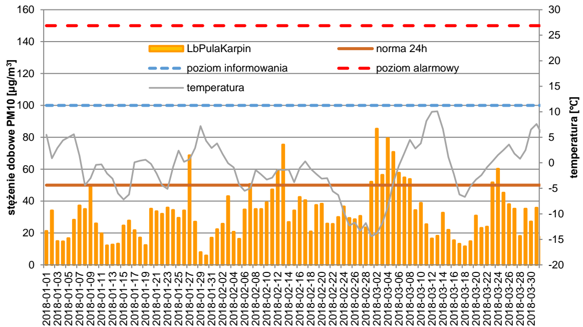
Rysunek 20. Porównanie przebiegu zmienności stężeń 24-godz. PM10 w I kwartale 2018 r. w Puławach z temperaturą
