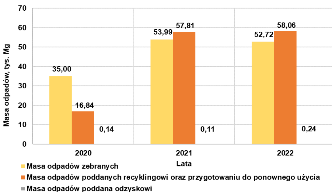
Rysunek 3.3.11 Masa zebranych odpadów w postaci zużytych opon w latach 2020-2022 59
